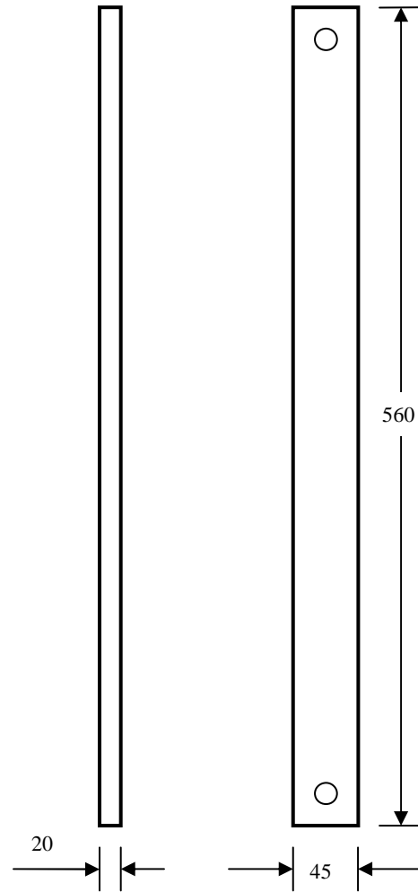
Aufhängeleiste – Teil 6
