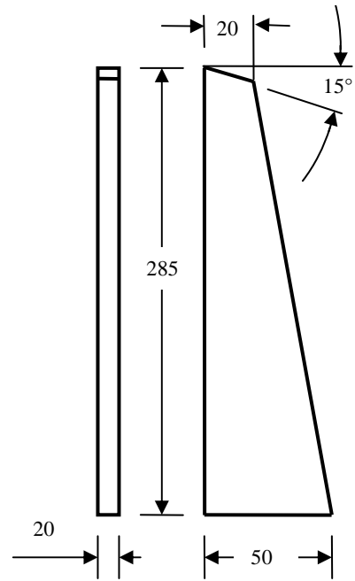
Seitenwand – Teil 5
